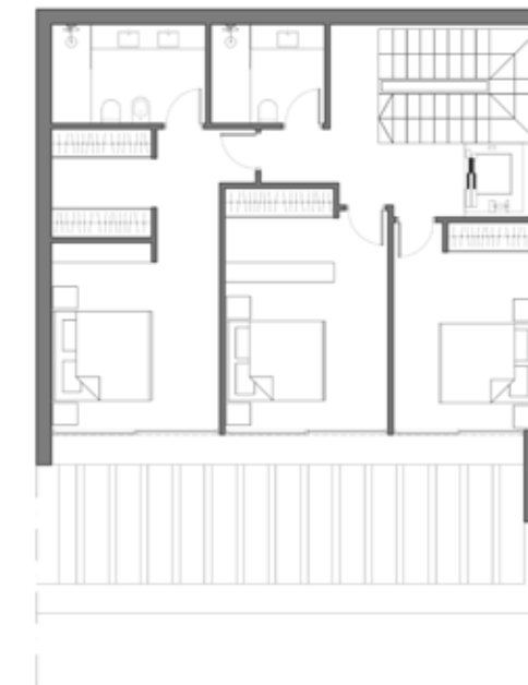
Primera planta
